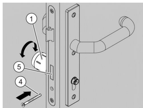
Afb. 62: De sluitneus positioneren
