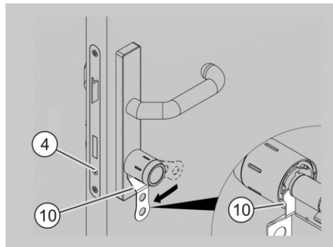
Afb. 107: De bajonetsluiting vergrendelen
