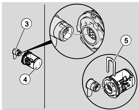
Afb. 128: De elektronische knop monteren
