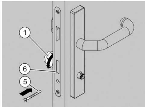
Afb. 13: De sluitneus positioneren
