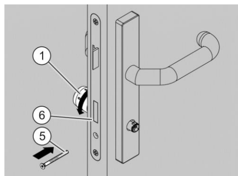
Afb. 88: De sluitneus positioneren
