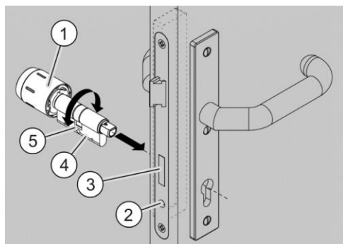
Afb. 97: De cilinder plaatsen
