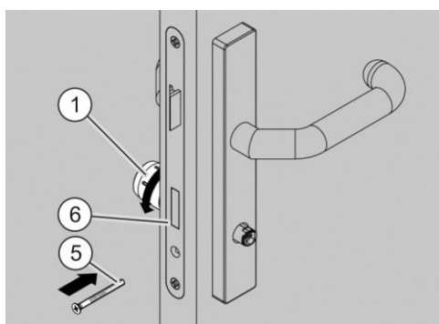
Afb. 54: De sluitneus positioneren
