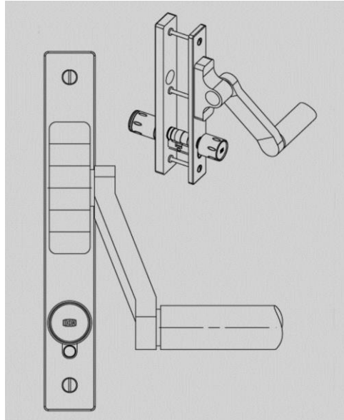
Afb. 76: Voorbeeld paniekstang
