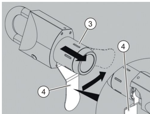
Afb. 163: De knophuls demonteren
