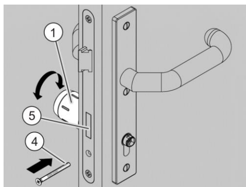
Afb. 31: De cilinder plaatsen
