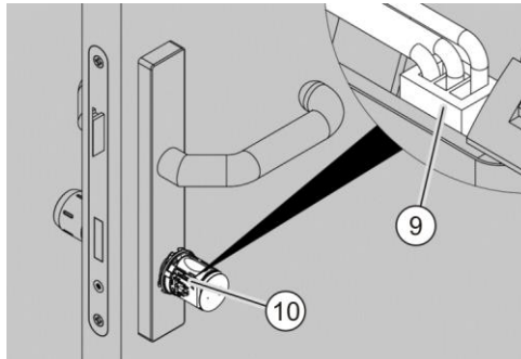
Afb. 56: De batterij aansluiten
