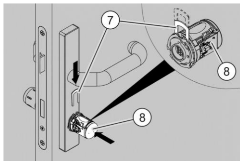
Afb. 14: De elektronische knop monteren
