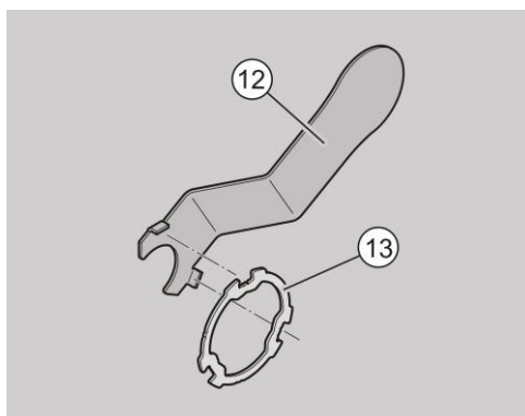
Afb. 58: Het knopgereedschap aanbrengen
