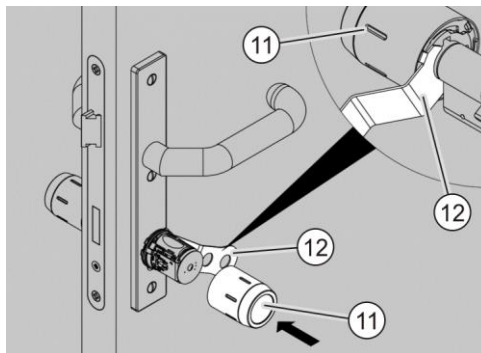
Afb. 57: De knophuls aanbrengen
