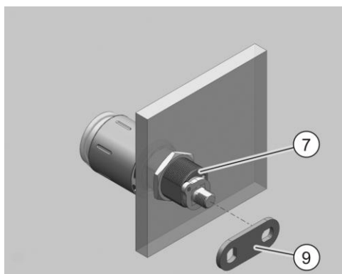
Afb. 145: De hevel aanbrengen
