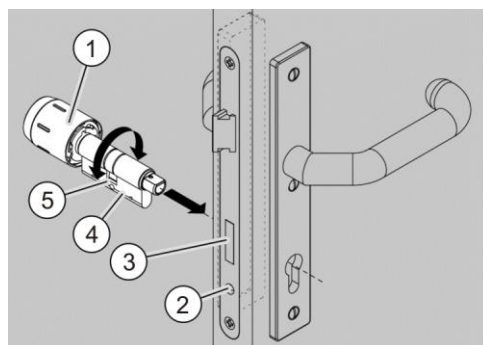
Afb. 111: De cilinder plaatsen
