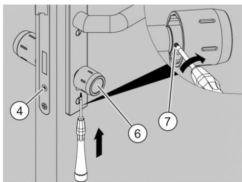
Afb. 65: De binnenknop bevestigen
