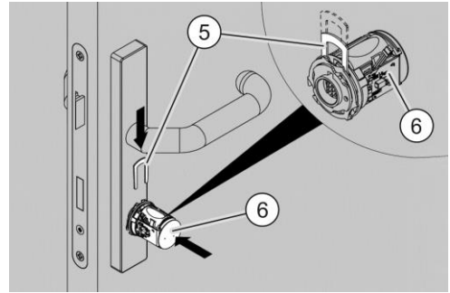
Afb. 24: De elektronische knop monteren
