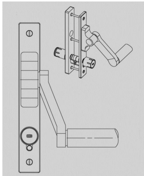
Afb. 83: Voorbeeld paniekstang
