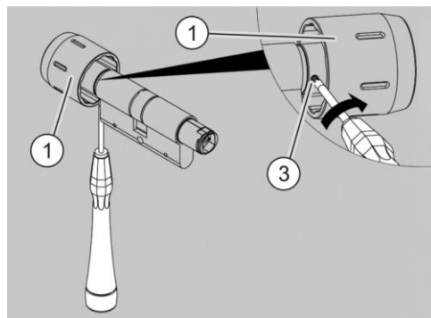
Afb. 86: De binnenknop vastdraaien
