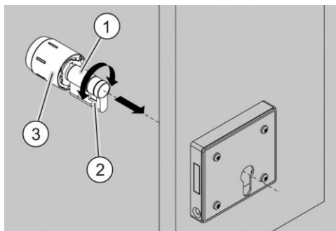
Afb. 124: De sluitneus positioneren
