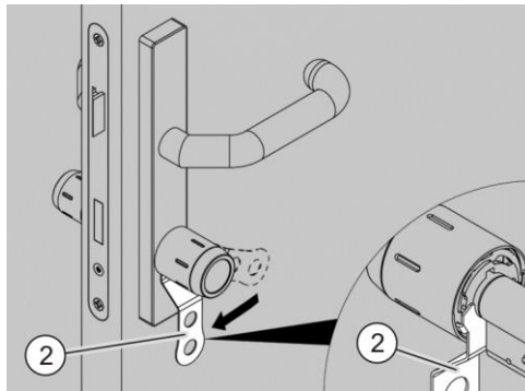
Afb. 160: De bajonetsluiting vergrendelen
