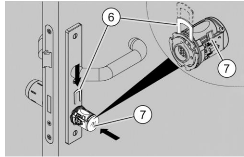
Afb. 40: De elektronische knop monteren
