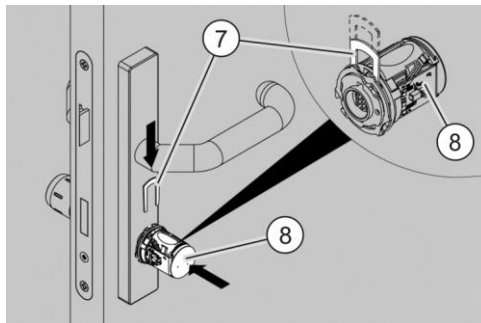
Afb. 89: De elektronische knop monteren
