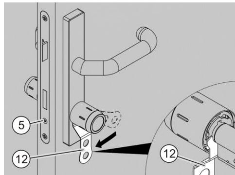
Afb. 75: De bajonetsluiting vergrendelen
