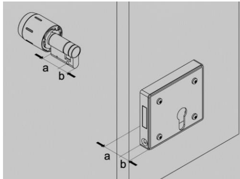
Afb. 123: De dikte meten
