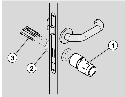
Afb. 148: De cilinder monteren
