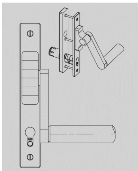
Afb. 99: Inbouwsituatie paniekstang
