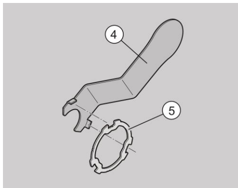
Afb. 164: Het knopgereedschap aanbrengen
