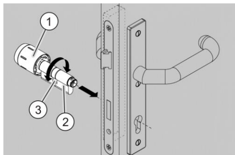
Afb. 38: De sluitneus positioneren
