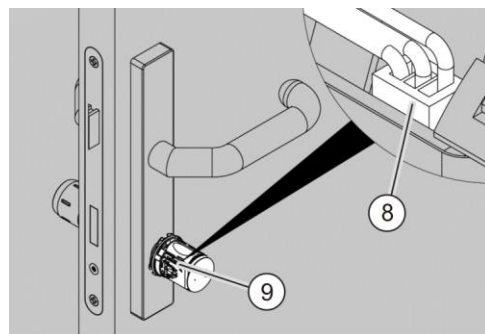
Afb. 33: De batterij aansluiten
