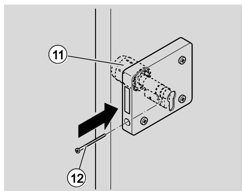
Afb. 133: De cilinder bevestigen
