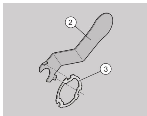
Afb. 159: Het knopgereedschap aanbrengen
