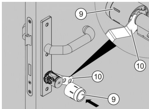
Afb. 26: De knophuls aanbrengen
