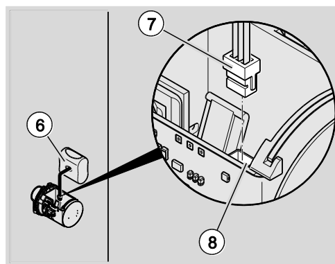
Afb. 129: De batterij aansluiten
