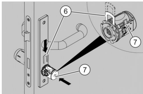
Afb. 32: De elektronische knop monteren
