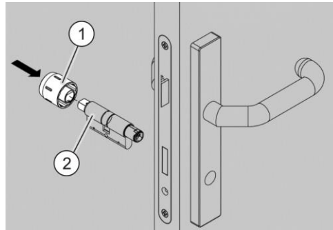
Afb. 85: De binnenknop aanbrengen
