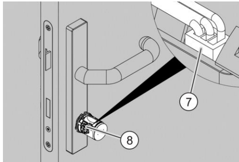
Afb. 25: De batterij aansluiten
