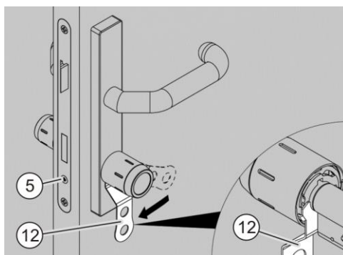
Afb. 93: De bajonetsluiting vergrendelen
