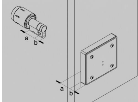
Afb. 134: De dikte meten
