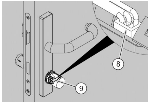
Afb. 41: De batterij aansluiten
