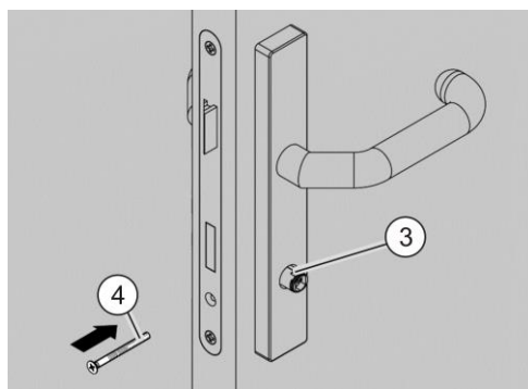
Afb. 102: De cilinder bevestigen
