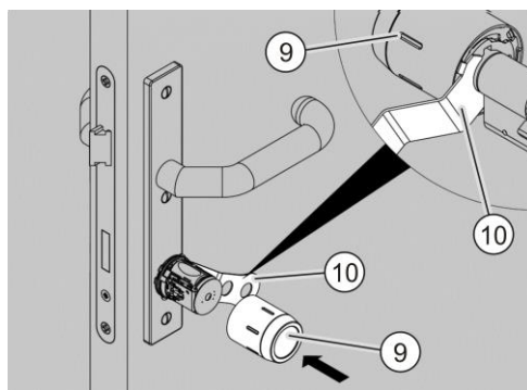
Afb. 105: De knophuls aanbrengen
