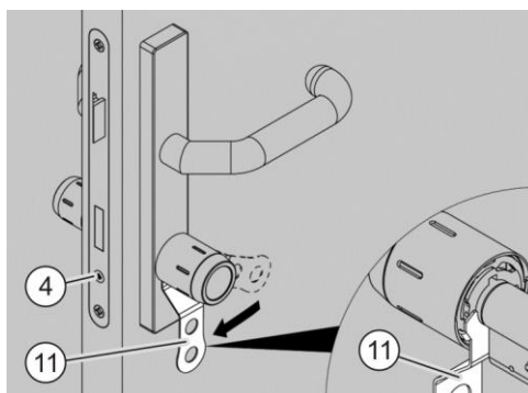
Afb. 36: De bajonetsluiting vergrendelen
