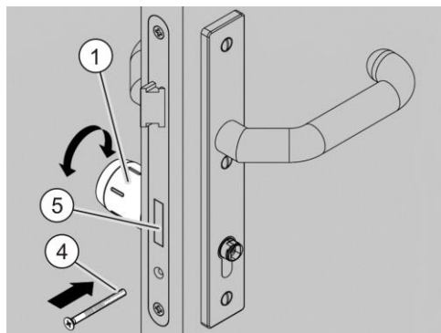
Afb. 47: De sluitneus positioneren
