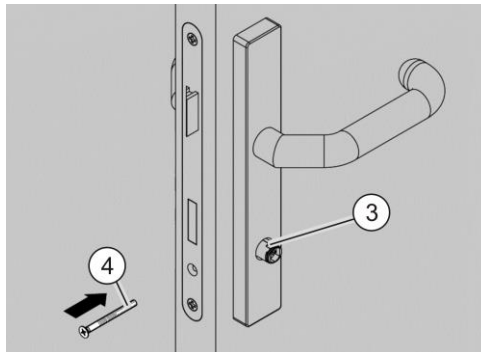
Afb. 116: De cilinder bevestigen
