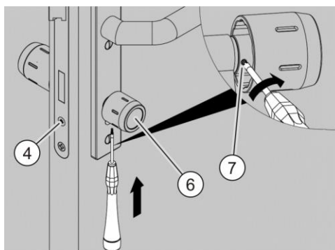
Afb. 49: De binnenknop bevestigen
