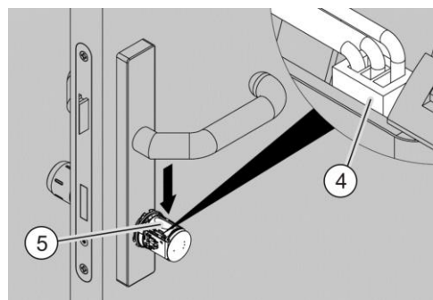
Afb. 157: Het batterijpack installeren
