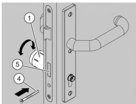
Afb. 39: De cilinder plaatsen
