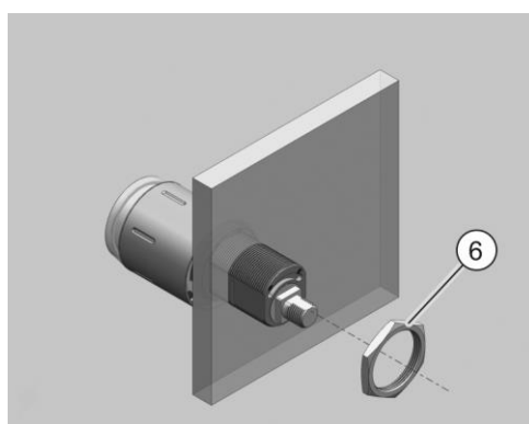
Afb. 141: De cilinder met de zeskantmoer bevestigen
