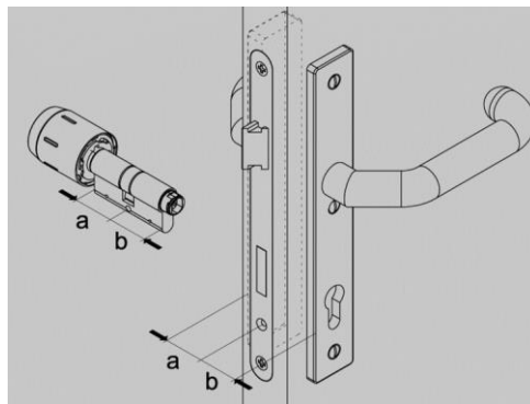
Afb. 4: De dikte meten
