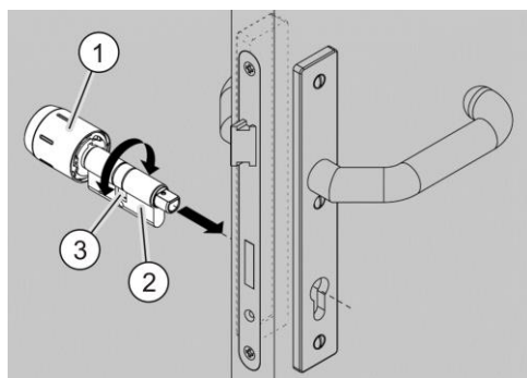
Afb. 78: De cilinder plaatsen
