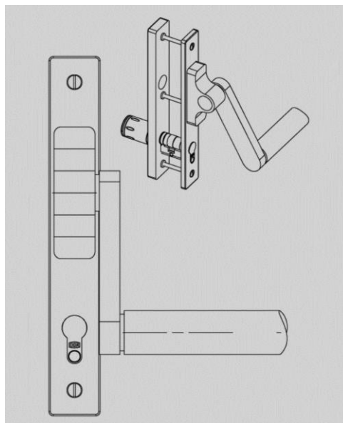
Afb. 95: Inbouwsituatie paniekstang
