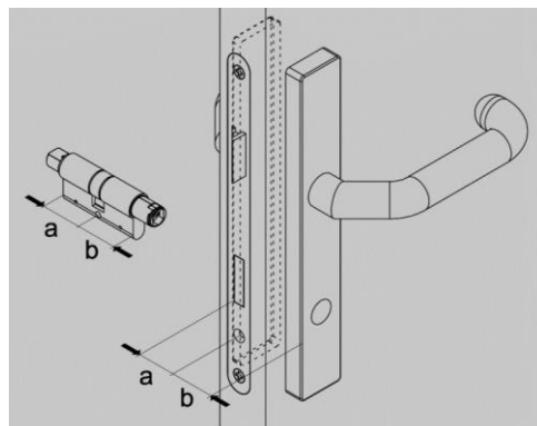
Afb. 100: De dikte meten
