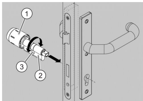
Afb. 5: De cilinder plaatsen
