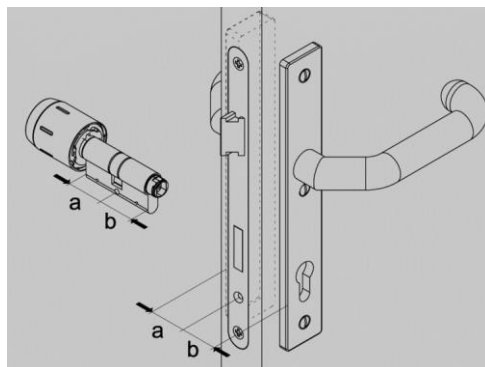
Afb. 96: De dikte meten
