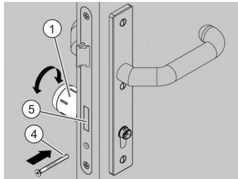
Afb. 6: De sluitneus positioneren
