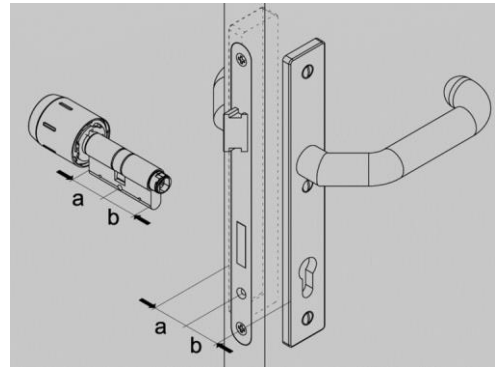
Afb. 19: De dikte meten
