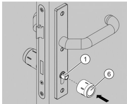
Afb. 7: De binnenknop aanbrengen
