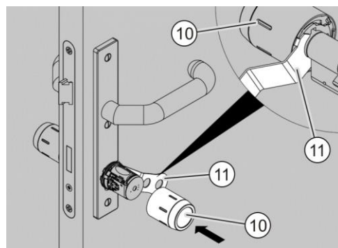
Afb. 34: De knophuls aanbrengen
