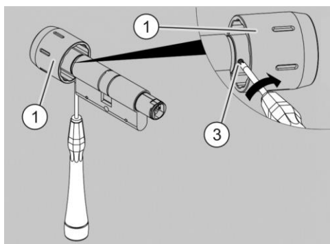
Afb. 68: De binnenknop vastdraaien
