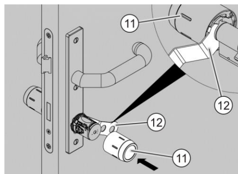
Afb. 91: De knophuls aanbrengen
