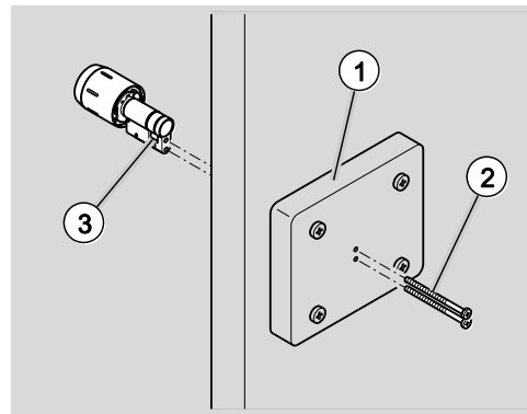
Afb. 135: De cilinder monteren
