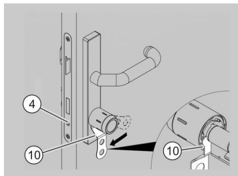
Afb. 121: De bajonetsluiting vergrendelen
